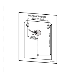
Gabarito de Instalação
